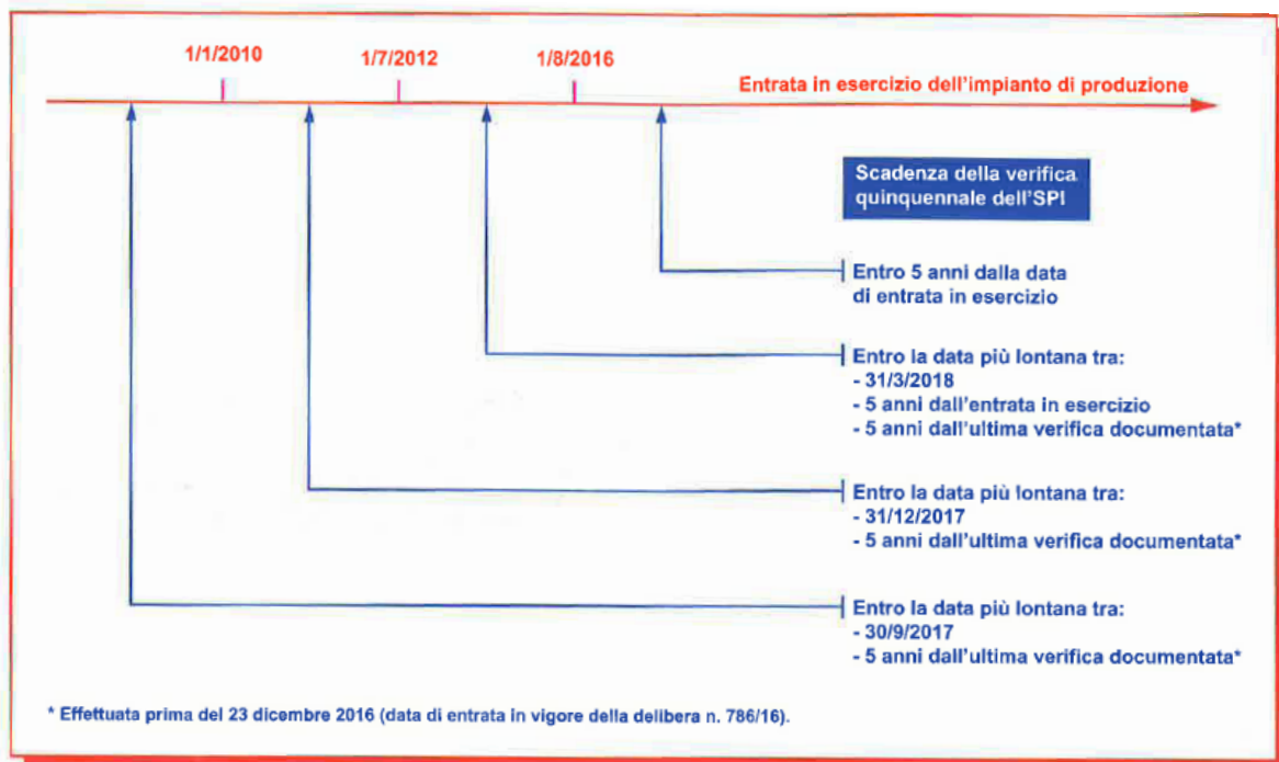
Fig. 1 - Scadenza della verifica quinquennale con la cassetta prova relè del sistema di protezione di interfaccia (utenti attivi, connessi in media tensione o in bassa tensione).
